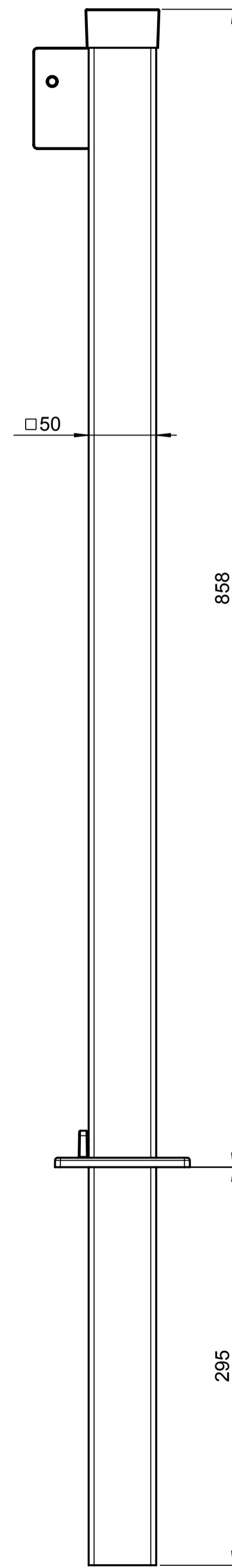
Einsteckpfosten SR414/2
